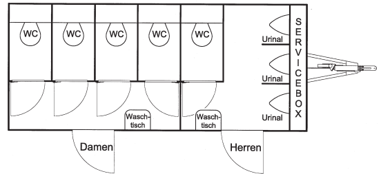
Raumeinteilung WC-Anhänger 5 m
